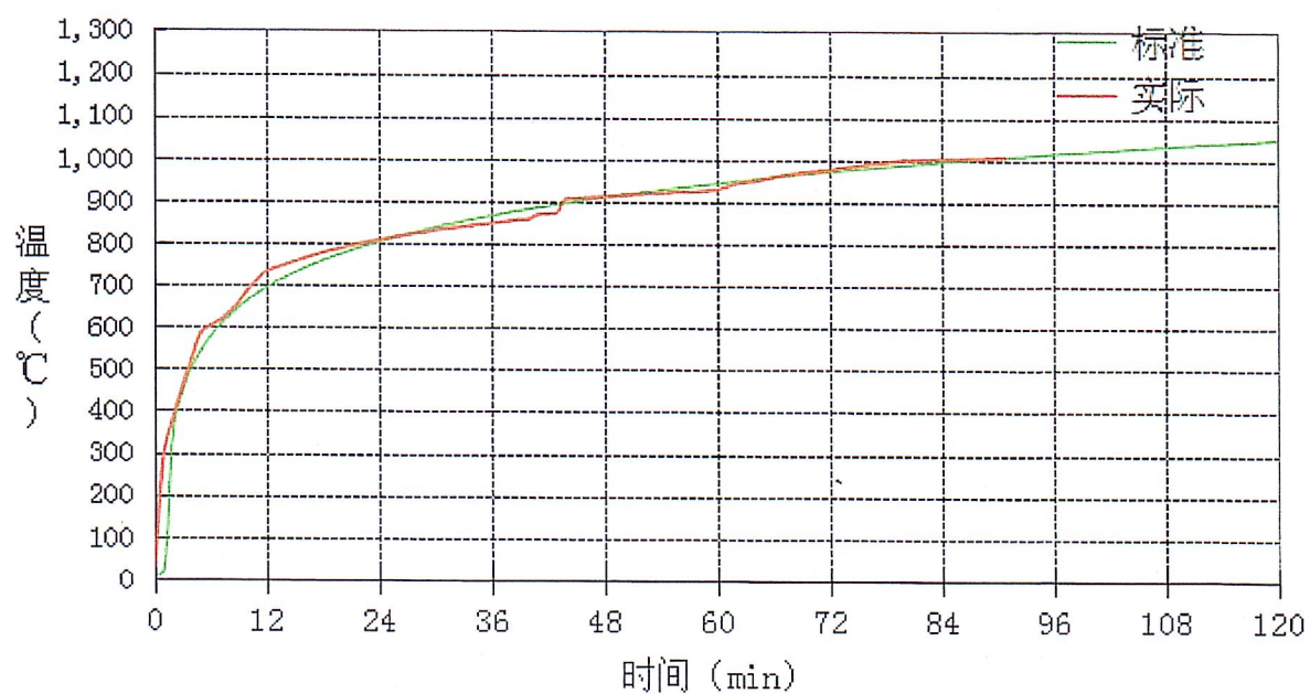
图1 炉内升温曲线
