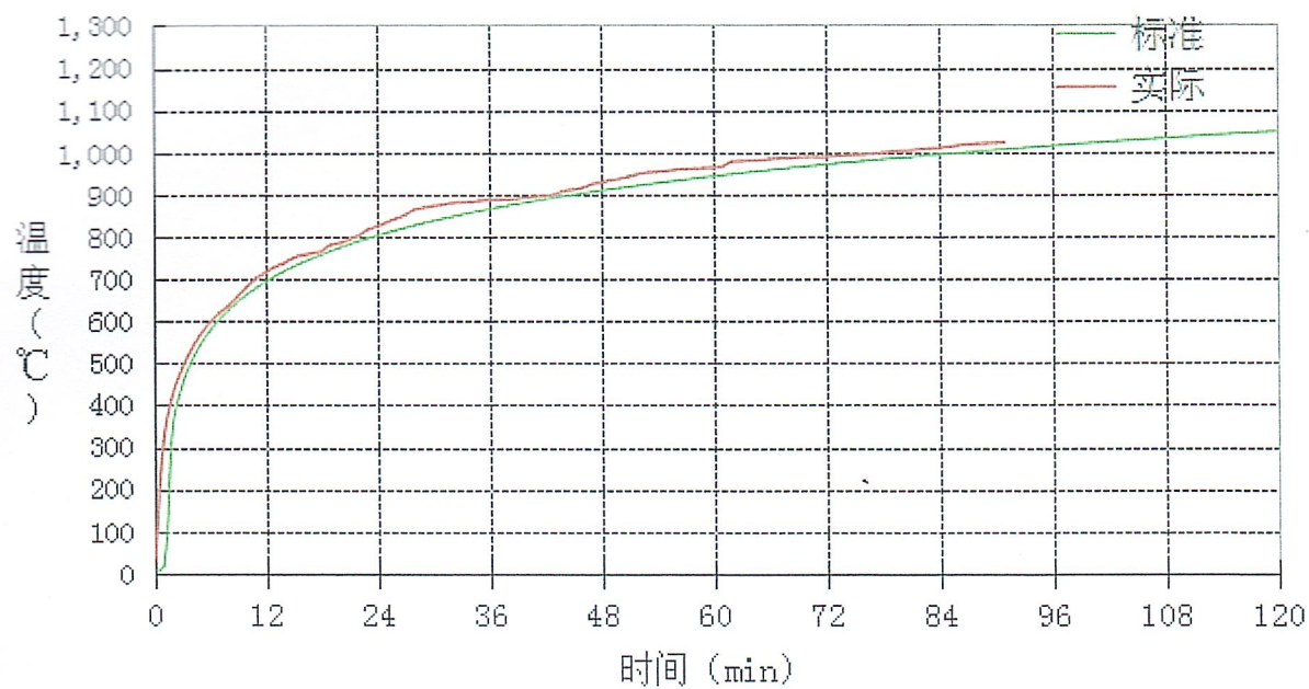
图1 炉内升温曲线
