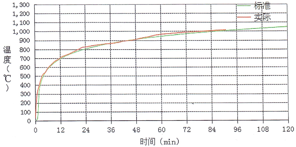
图1 炉内升温曲线
